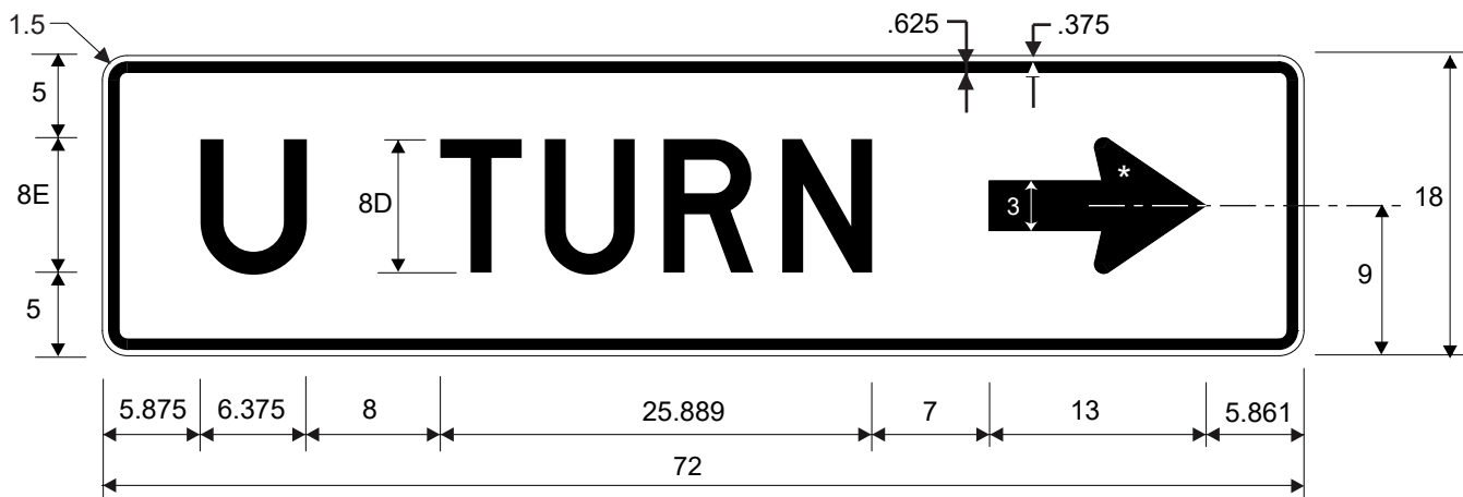
R3-25b U TURN (Arrow)
