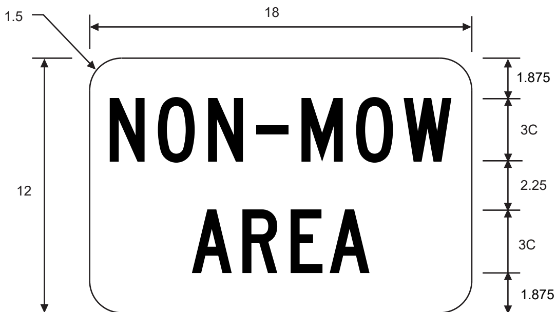
R19-11T NON-MOW AREA
